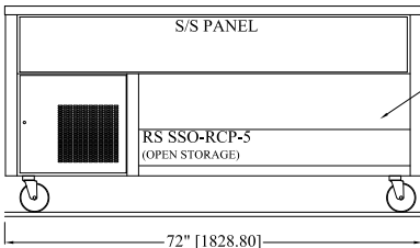
RS SSC-RCP-5 PANEL IN LIEU OF SHELF (ENCLOSED BASE) RS SSO-RCP-5 (OPEN STORAGE)
