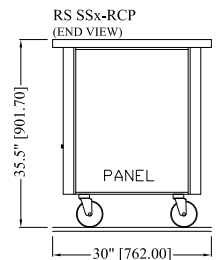
RS SSC-RCP-6 PANEL IN LIEU OF SHELF (ENCLOSED BASE) RS SSO-RCP-6 (OPEN STORAGE)
