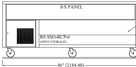
RS SSC-RCP-6 PANEL IN LIEU OF SHELF (ENCLOSED BASE) RS SSO-RCP-6 (OPEN STORAGE)
